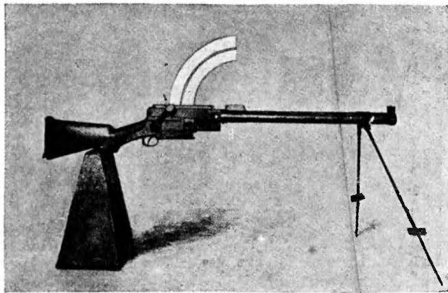
Усовершенствованная митральеза. Ружье Рексера, приготовленное к стрельбе.
